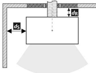
Hátsó kéménycsatlakozás
