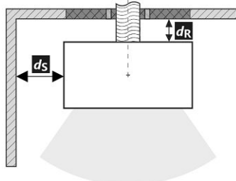
Zadní napojení kouřovodu
