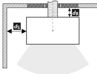
Hátsó kéménycsatlakozás
