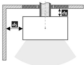
Tylne przyłącze kominowe (izolowane)
